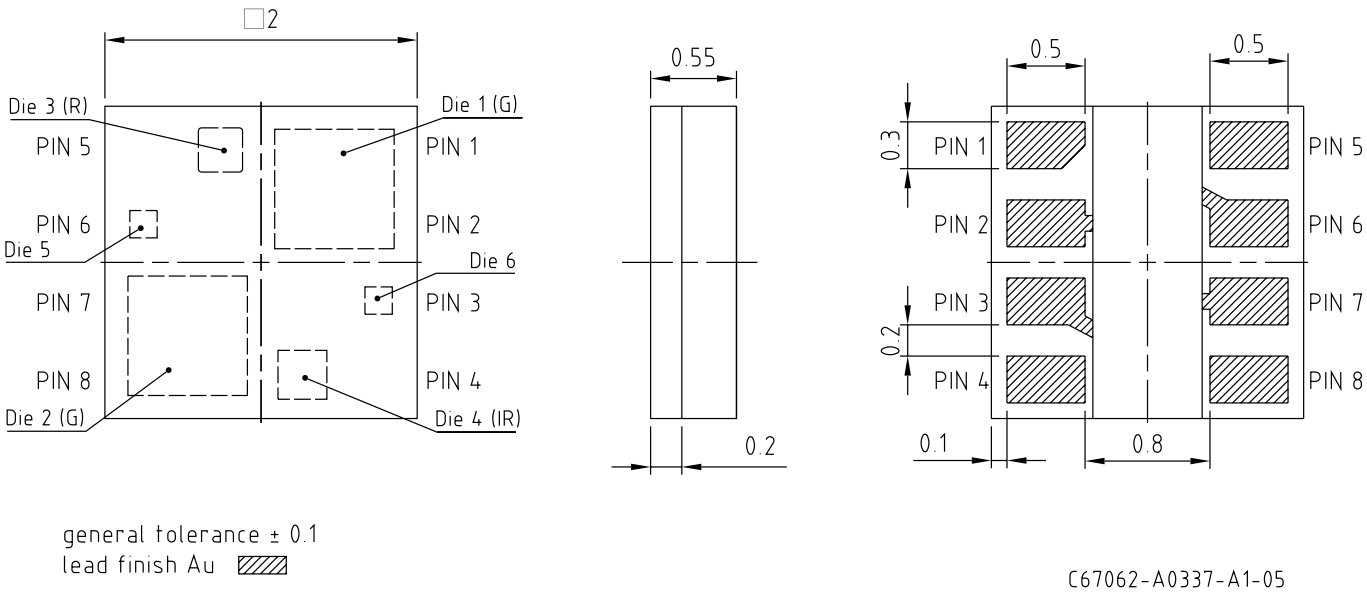
尺寸图 10)
