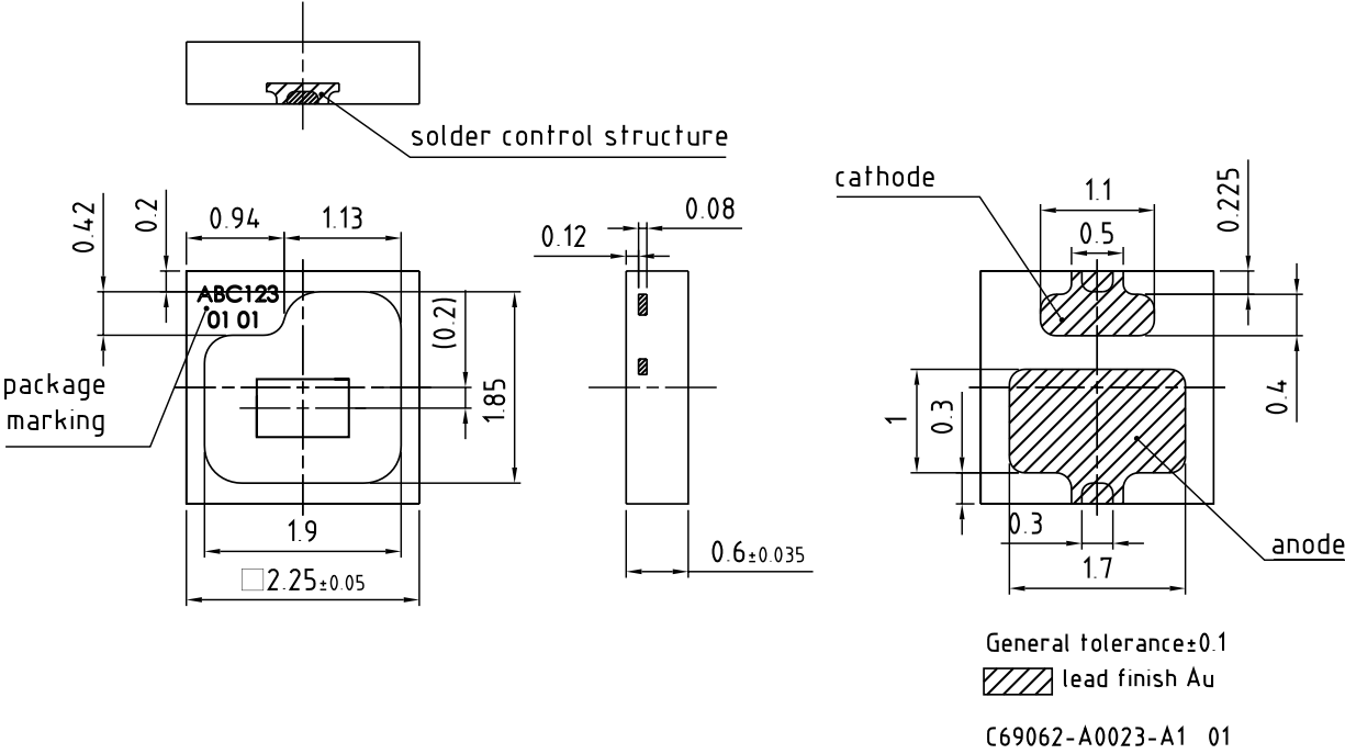
尺寸图 9)
