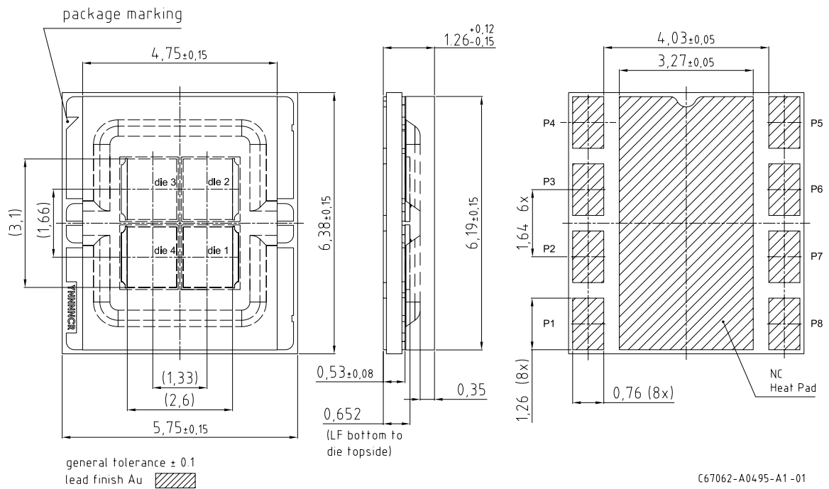
尺寸图 8)
