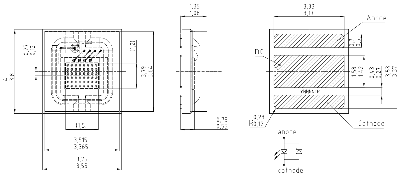
尺寸图 8)
