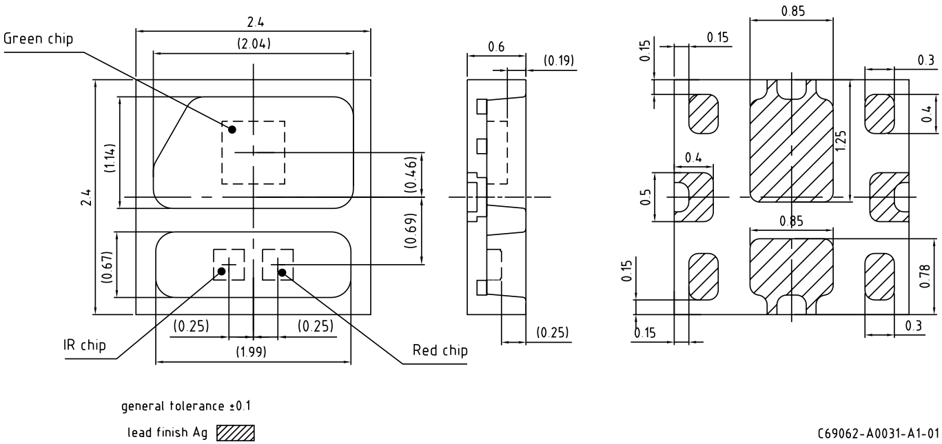
尺寸图 10)
